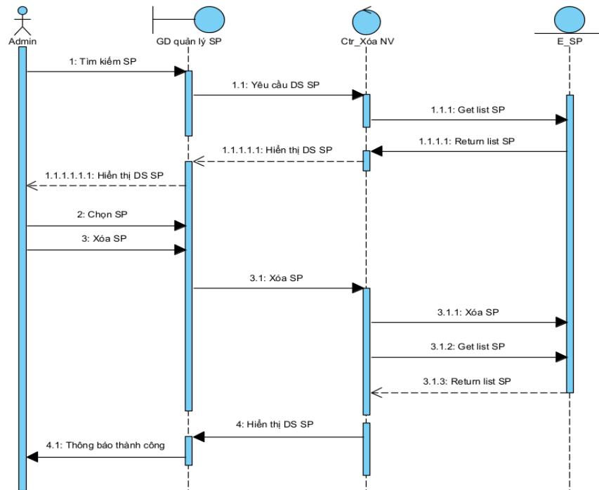
Hình 3-14 Biểu đồ tuần tự xóa sản phẩm
