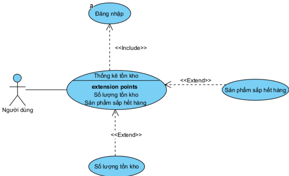
Hình 3-9 Usecase phân rã chức năng thống kê tồn kho
