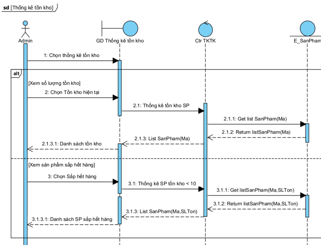
Hình 3-27 Biểu đồ tuần tự thống kê tồn kho
