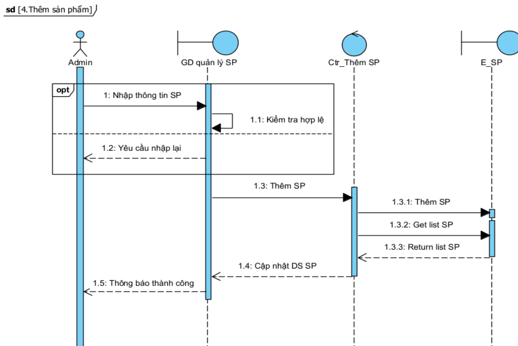
Hình 3-12 Biểu đồ tuần tự thêm sản phẩm
