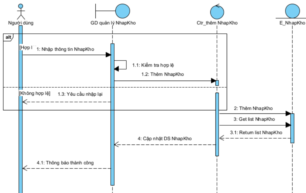
Hình 3-21 Biểu đồ tuần tự thêm phiếu nhập kho
