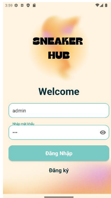
Hình 4-1 Chức năng Đăng nhập
