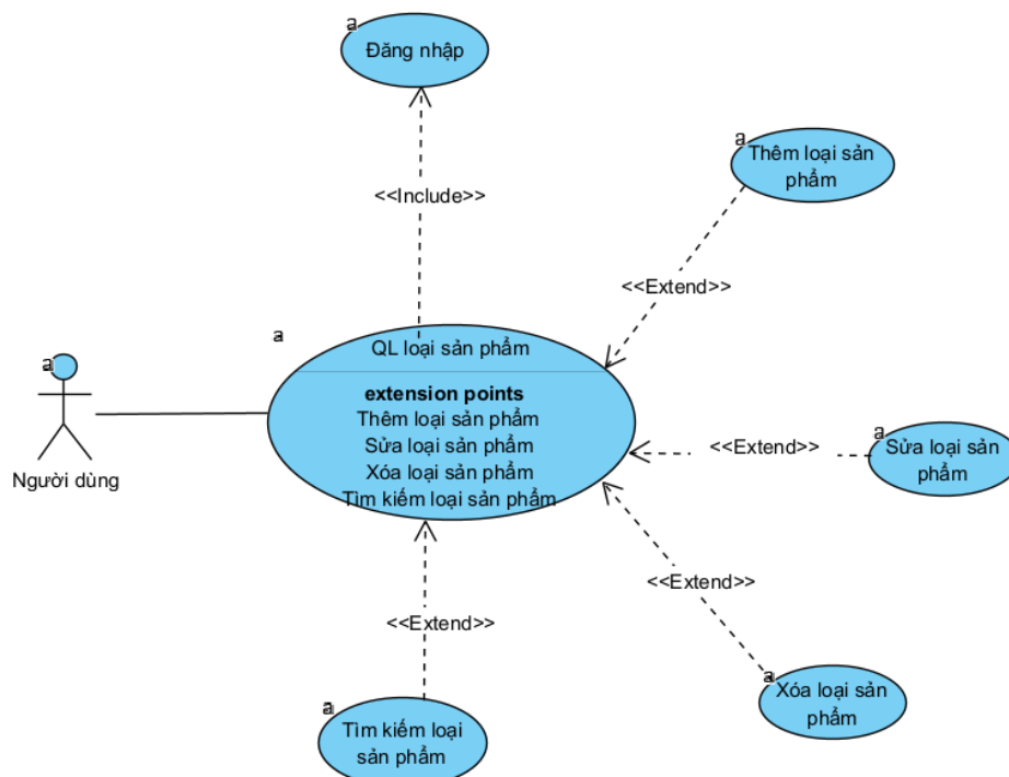
Hình 3-5 Usecase chức năng Quản lý loại sản phẩm
