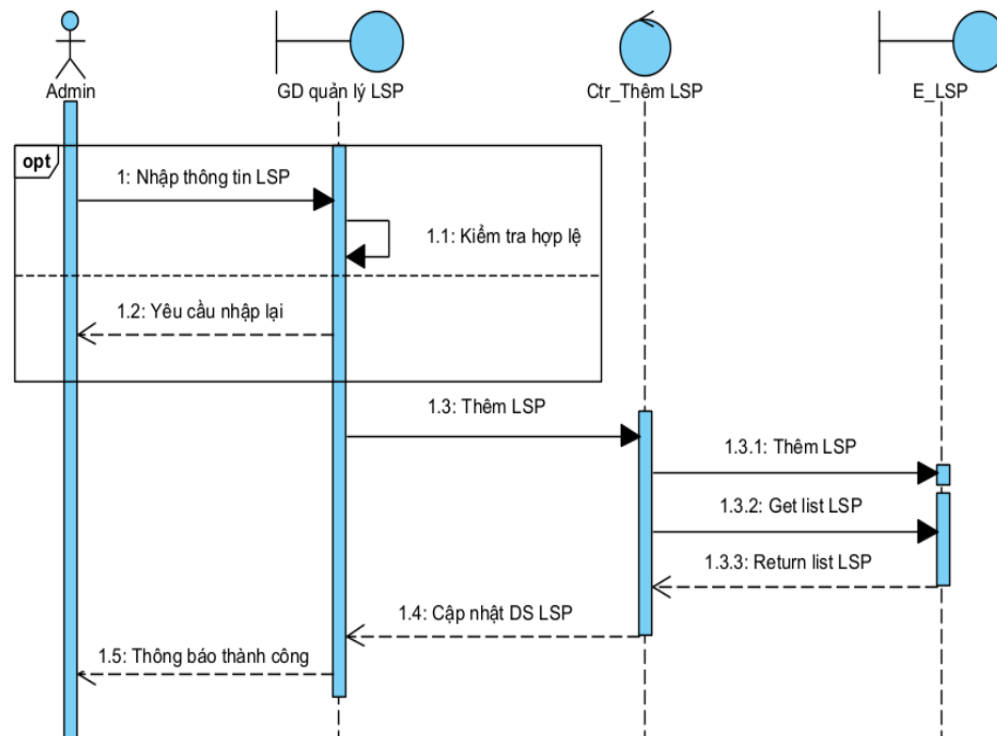
Hình 3-15 Biểu đồ tuần tự thêm loại sản phẩm
