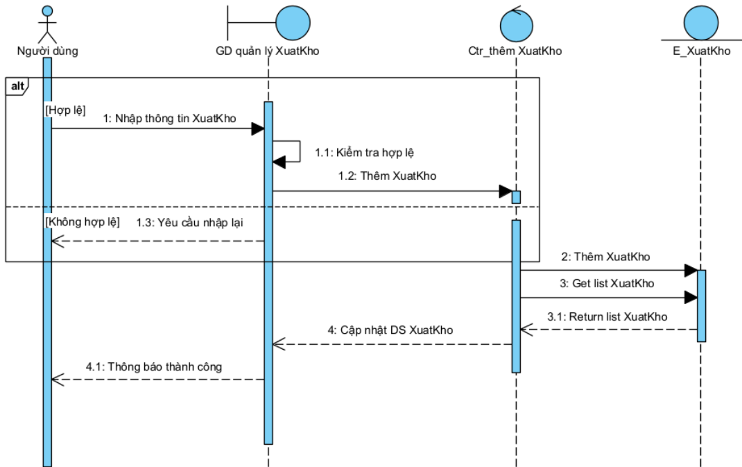
Hình 3-24 Biểu đồ tuần tự thêm phiếu xuất kho
