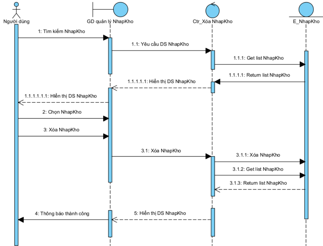
Hình 3-23 Biểu đồ tuần tự xóa phiếu nhập kho
