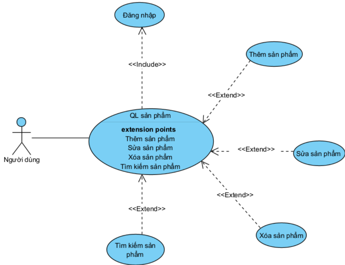
Hình 3-4 Usecase chức năng Quản lý sản phẩm
