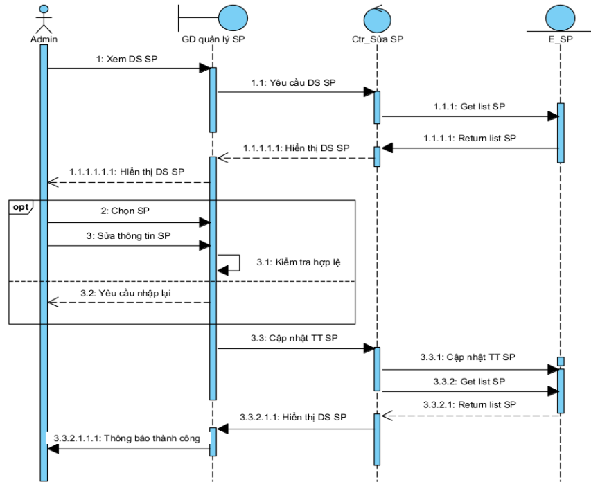
Hình 3-13 Biểu đồ tuần tự sửa sản phẩm
