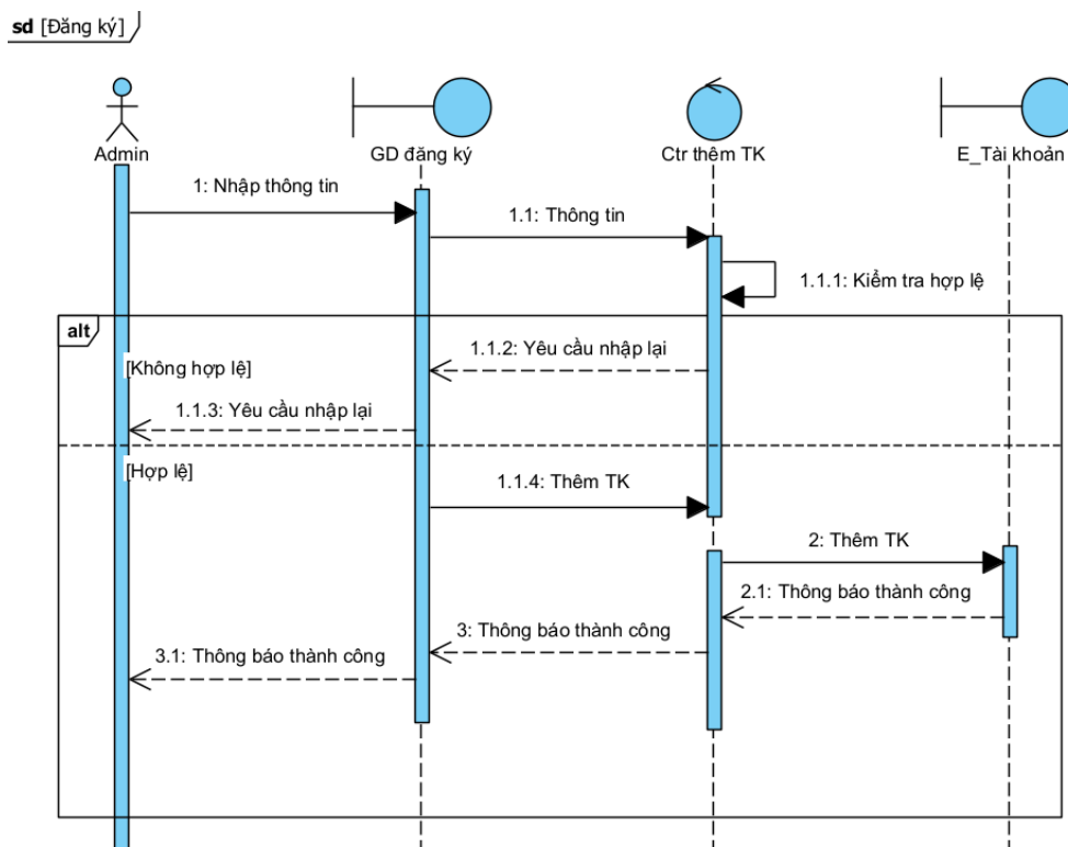
Hình 3-11 Biểu đồ tuần tự đăng ký
