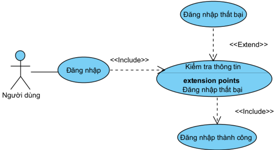
Hình 3-2 Usecase phân rã chức năng đăng nhập
