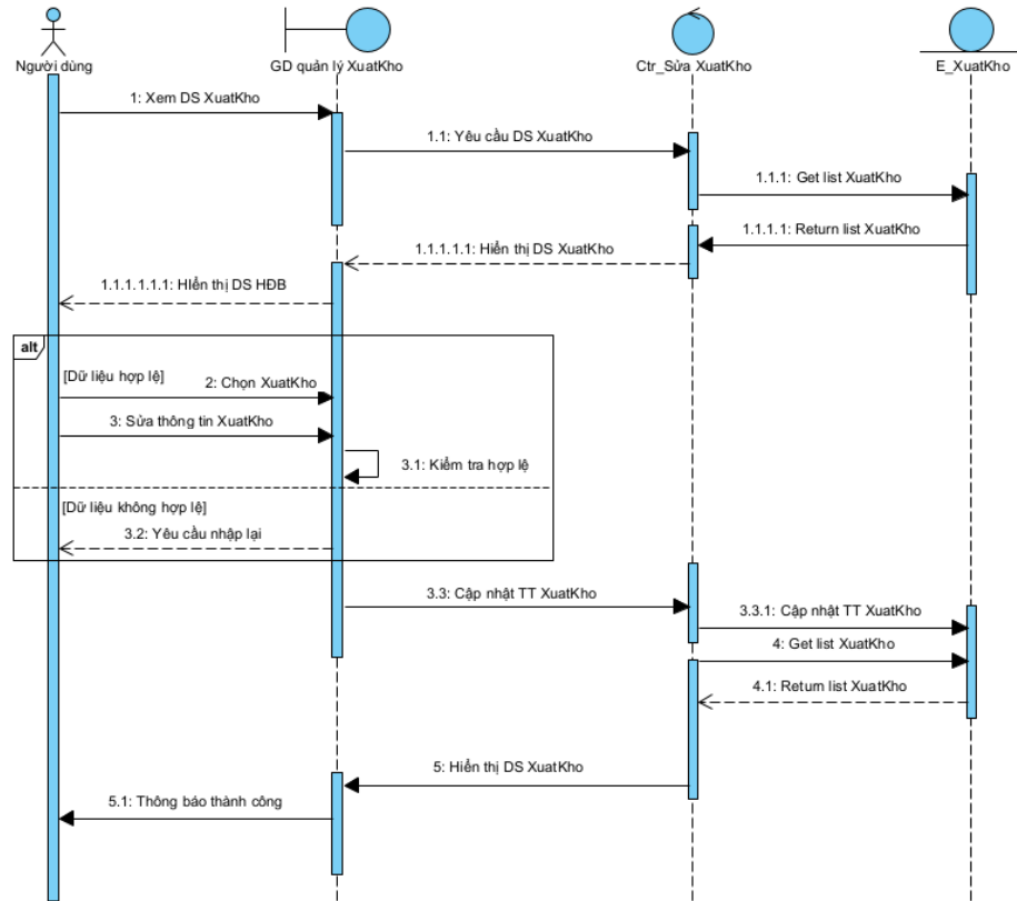
Hình 3-25 Biểu đồ tuần tự sửa phiếu xuất kho
