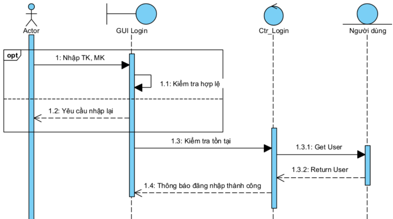
Hình 3-10 Biểu đồ tuần tự đăng nhập
