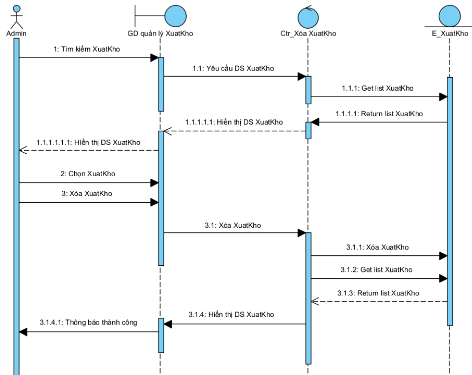
Hình 3-26 Biểu đồ tuần tự xóa phiếu xuất kho
