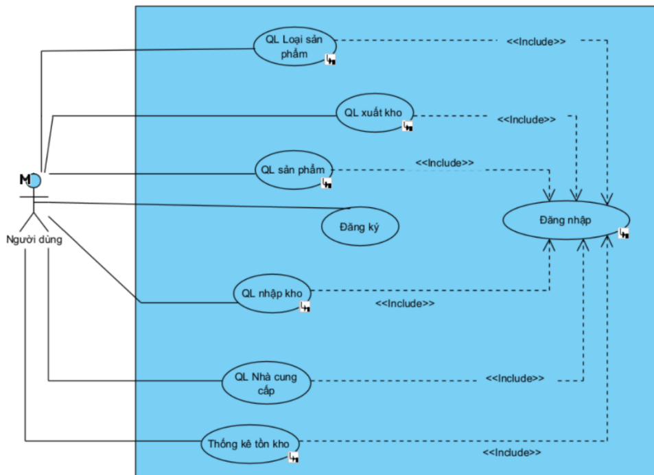
Hình 3-1 Usecase tổng quát
