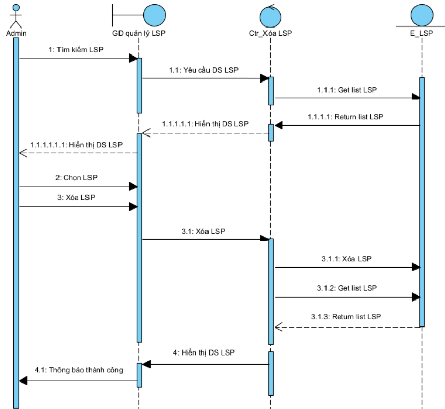
Hình 3-17 Biểu đồ tuần tự xóa loại sản phẩm
