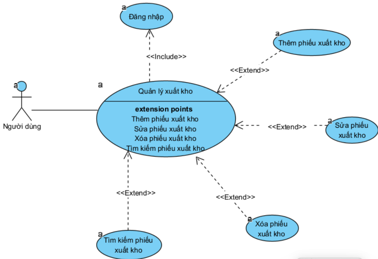
Hình 3-8 Usecase chức năng Quản lý xuất kho
