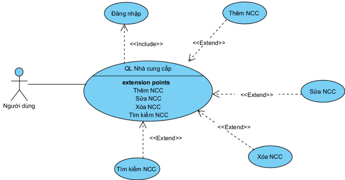
Hình 3-6 Usecase chức năng Quản lý nhà cung cấp
