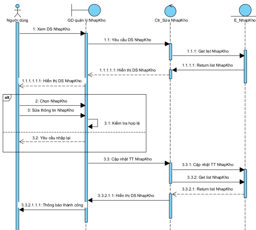
Hình 3-22 Biểu đồ tuần tự sửa phiếu nhập kho
