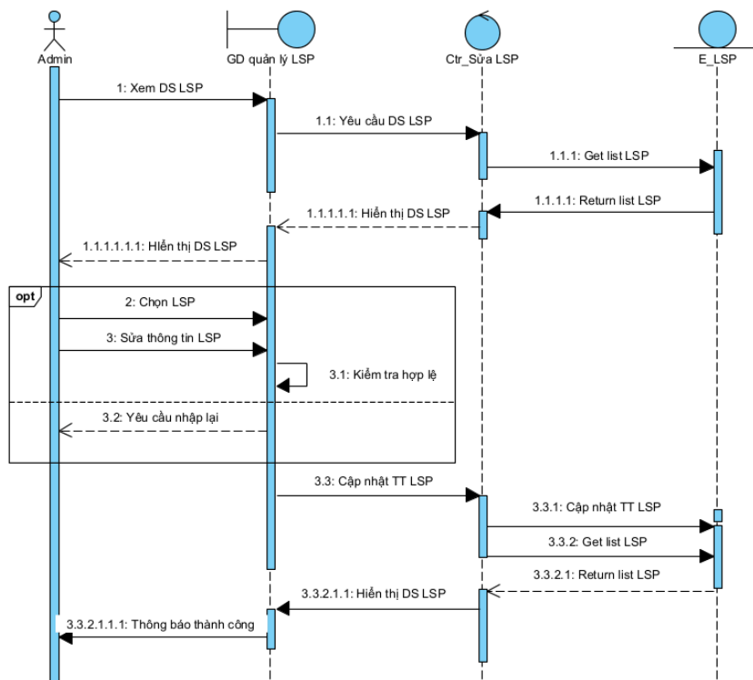
Hình 3-16 Biểu đồ tuần tự sửa loại sản phẩm
