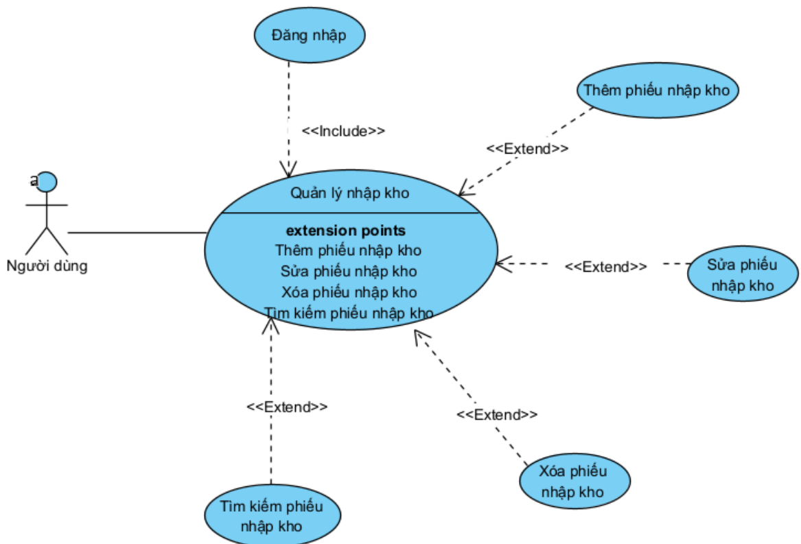
Hình 3-7 Usecase chức năng Quản lý nhập kho
