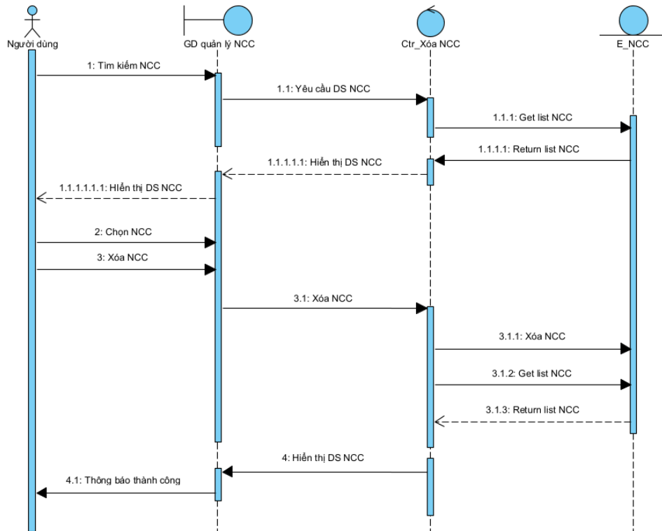
Hình 3-20 Biểu đồ tuần tự xóa nhà cung cấp
