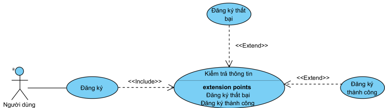
Hình 3-3 Usecase chức năng Đăng ký
