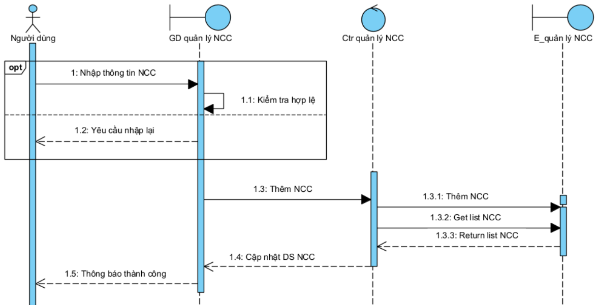
Hình 3-18 Biểu đồ tuần tự thêm nhà cung cấp
