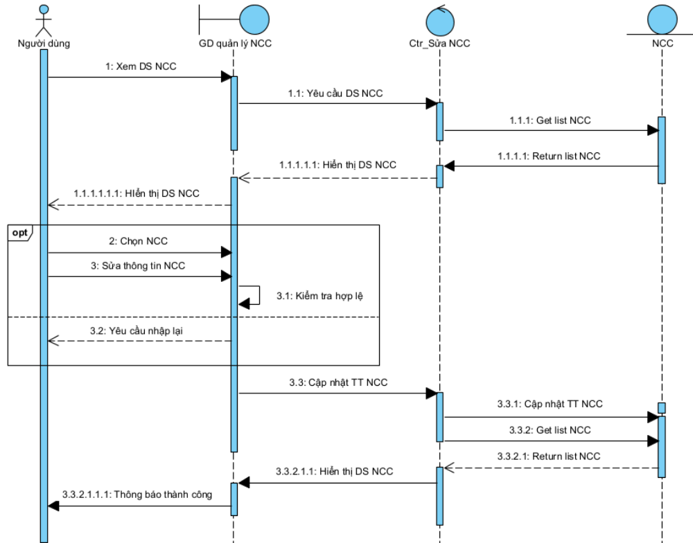
Hình 3-19 Biểu đồ tuần tự sửa nhà cung cấp
